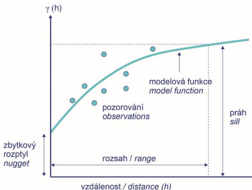
Obr. 19 Diagram znázorňující parametry variogramu a proloženou sférickou křivku
