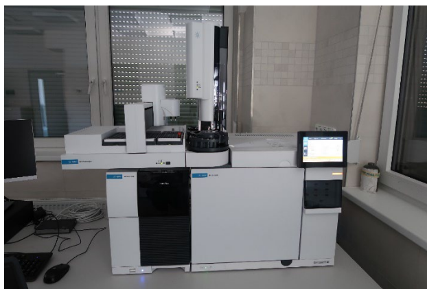
Obr. 11 Plynový chromatograf s chemickou ionizací, na kterém je vyvíjena metoda pro stanovení nitro-PAH (P-ČHMÚ Ústí nad Labem)
